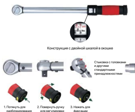
1. Погнуть для разблокирования 2. Повернуть ручку для регулировки момента 3. Нажать для фиксации
